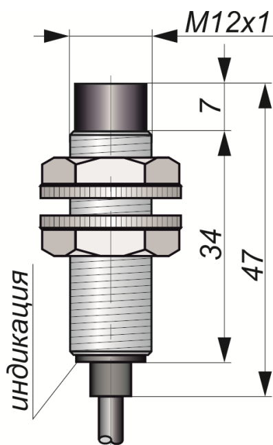
Габаритный чертеж
